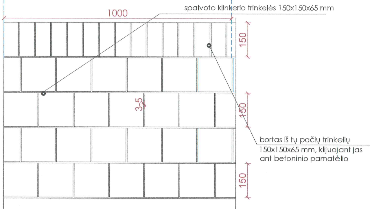
KLOJIMO RAŠTAS TAKUOSE spalvoto klinkerio trinkelės 150x150x65 mm
